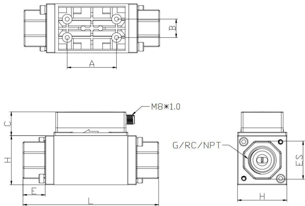
图8. MS-FX40系列外形尺寸图（单位：mm，L公差：±1mm,其余未标公差：±0.5
